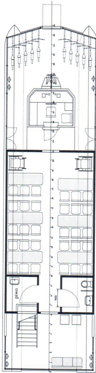
pokład główny - 32 miejsca siedzące
