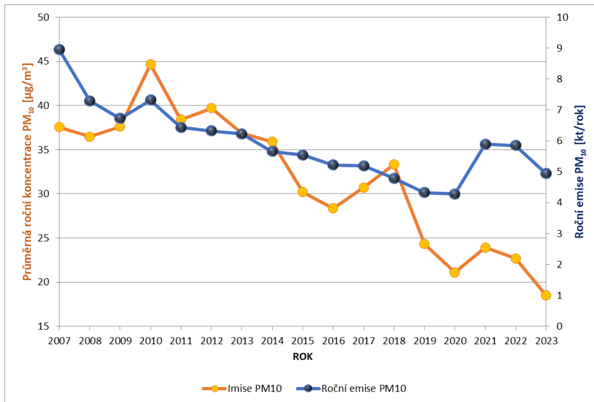
Obrázek 56 - Vyobrazení emisně - imisních vztahů pro PM 10
