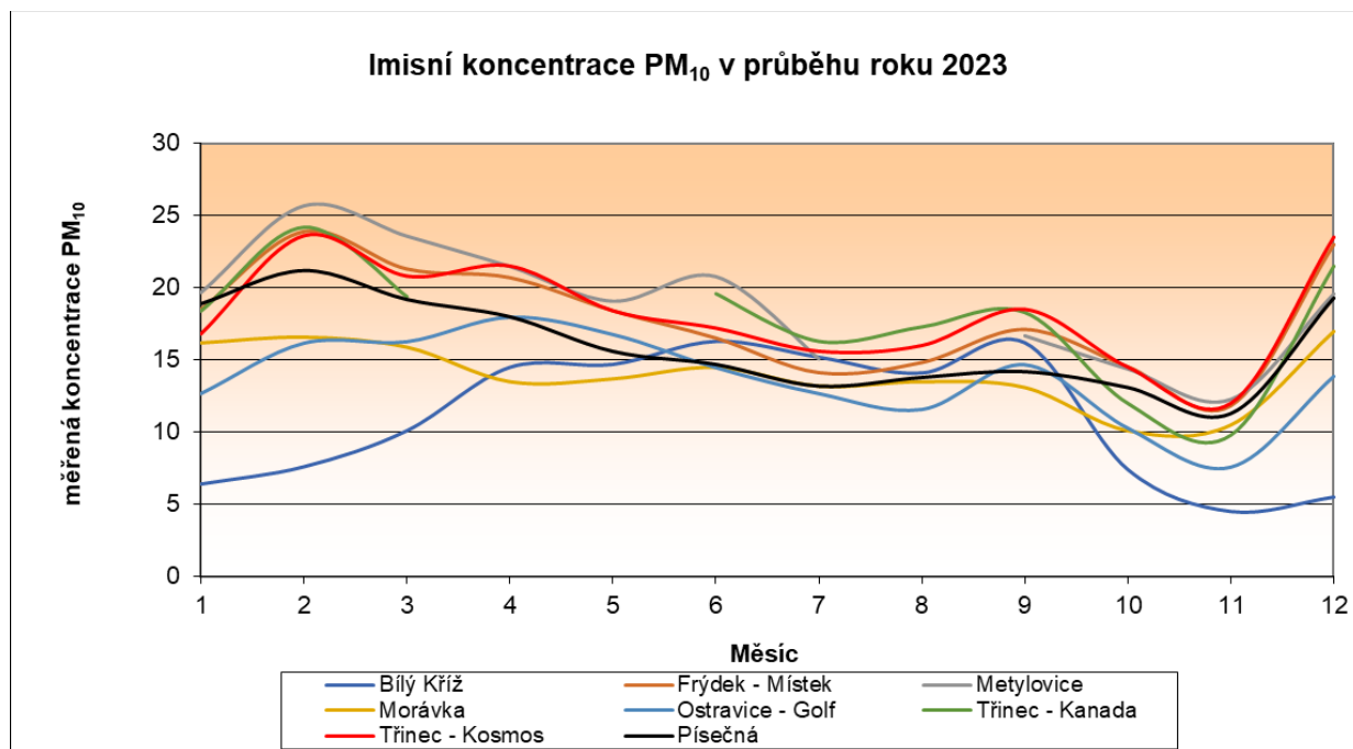
Obrázek 21 Roční chod imisních koncentrací PM 10 v roce 2023 [μg/m 3 ] Okres Frýdek – Místek
