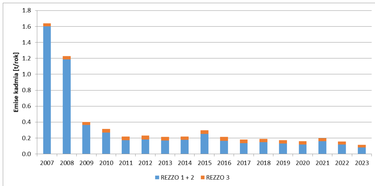
Obrázek 13 - Emise kadmia jednotlivých skupin zdrojů v MSK
