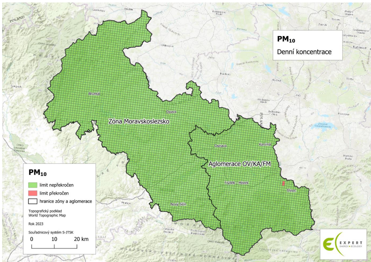
Obrázek 43 - Oblasti s překročením imisního limitu pro denní koncentrace PM 10 - rok 2023
