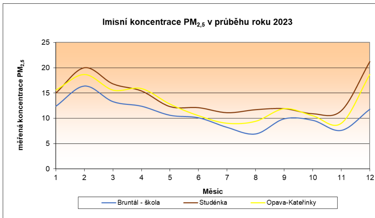
Obrázek 28 Roční chod imisních koncentrací PM 2,5 v roce 2023 [µg/m 3 ]
