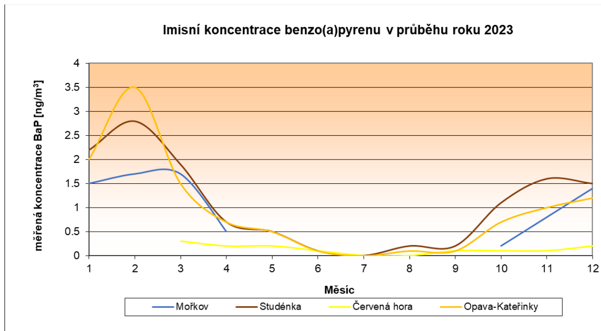
Obrázek 37 Roční chod imisních koncentrací benzo(a)pyrenu v roce 2023 [ng/m 3 ] Okresy Opava, Nový Jičín
