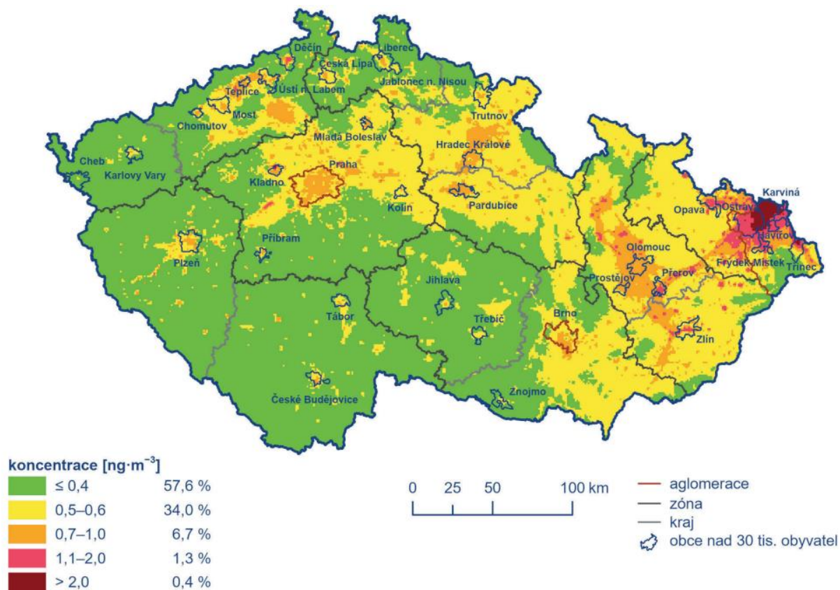
Obrázek 41 - Pole roční průměrné koncentrace benzo(a)pyrenu v ovzduší v roce 2023
