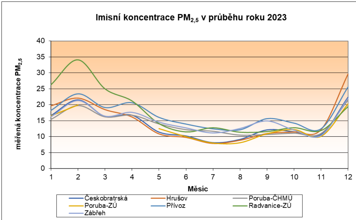
Obrázek 31 Roční chod imisních koncentrací PM 2,5 v roce 2023 [µg/m 3 ] Okres Ostrava
