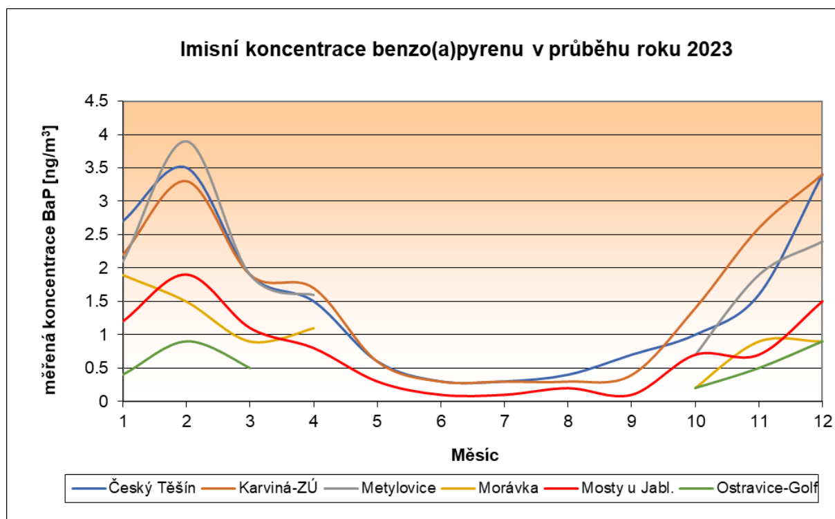
Obrázek 38 Roční chod imisních koncentrací benzo(a)pyrenu v roce 2023 [ng/m 3 ] Okres Karviná, Frýdek-Místek
