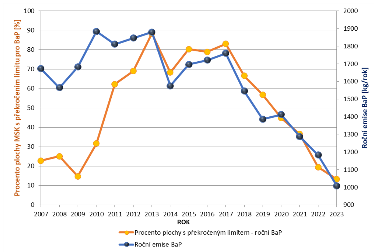
Obrázek 61 - Vyobrazení plochy s překročeným limitem a emisí BaP v historických datech
