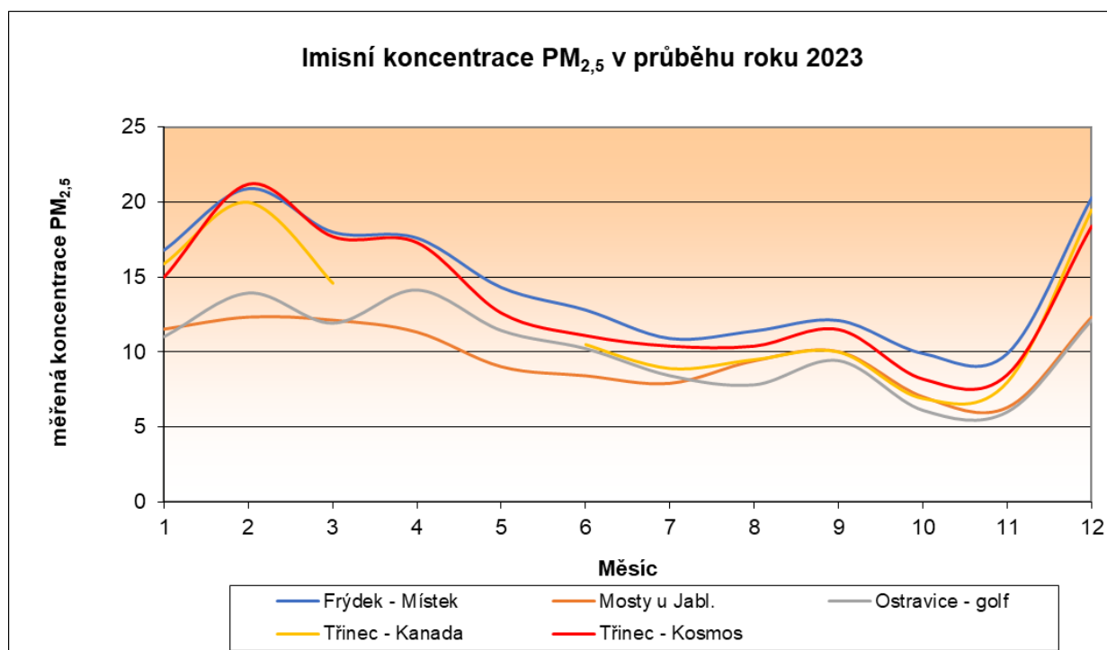
Obrázek 29 Roční chod imisních koncentrací PM 2,5 v roce 2023 [µg/m 3 ] Okres Frýdek-Místek
