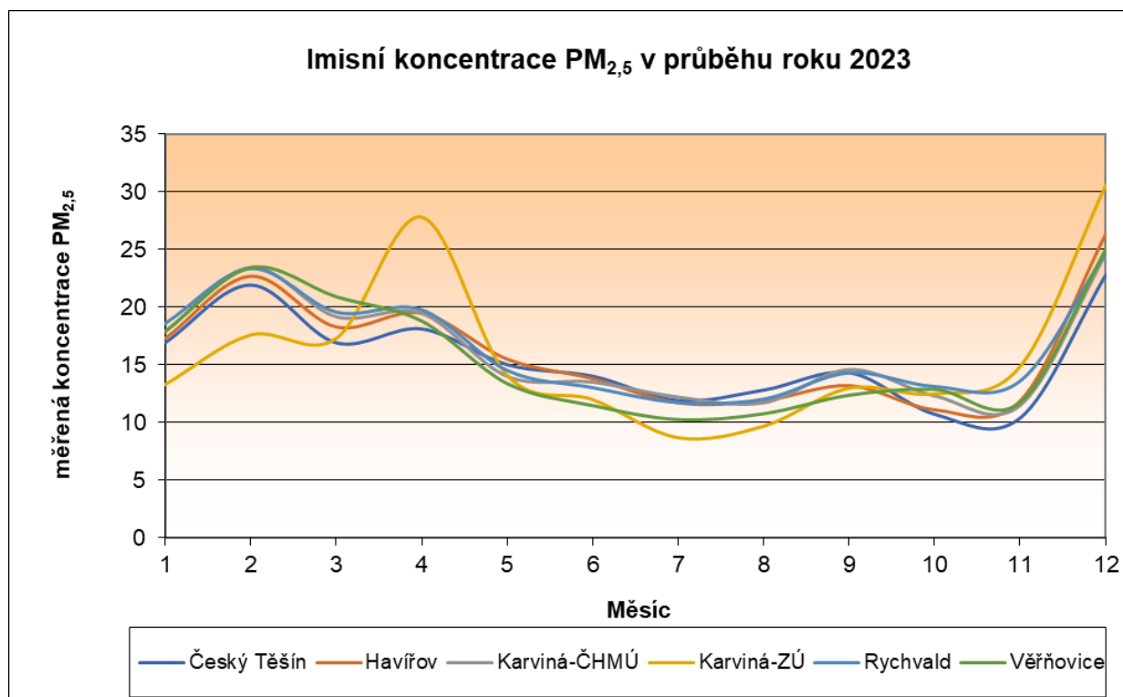
Obrázek 30 Roční chod imisních koncentrací PM 2,5 v roce 2023 [µg/m 3 ] Okres Karviná
