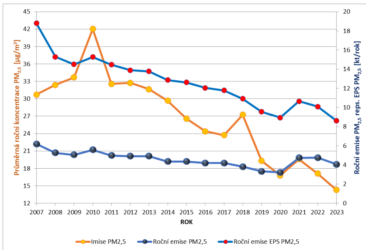
Obrázek 58 - Vyobrazení emisně - imisních vztahů pro PM 2,5
