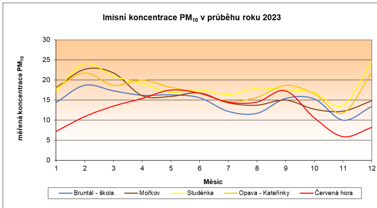
Obrázek 20 Roční chod imisních koncentrací PM 10 v roce 2023 [μg/m 3 ] okresy Nový Jičín, Opava, Bruntál
