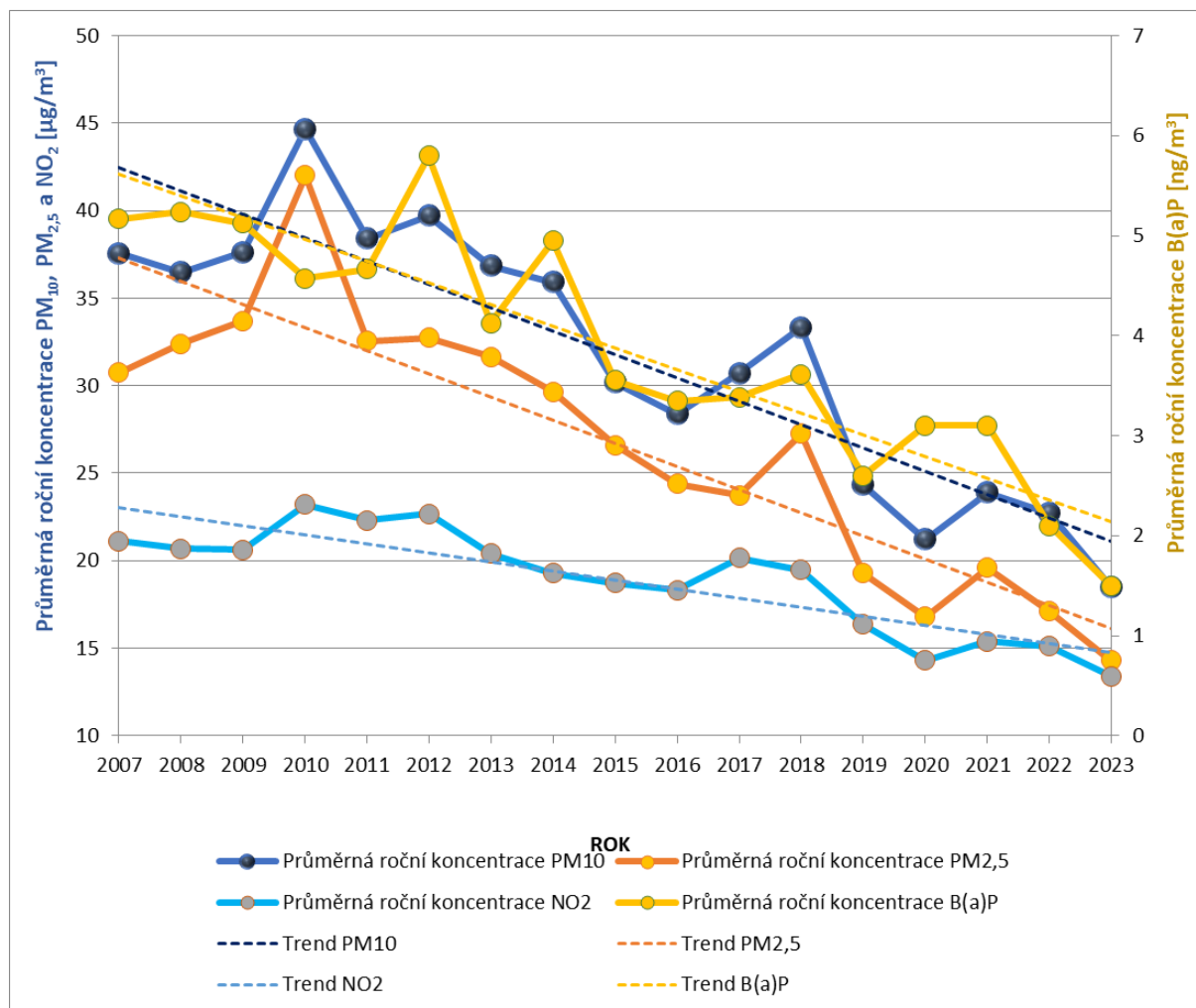
Obrázek 63 - Trendy imisí hlavních škodlivin
