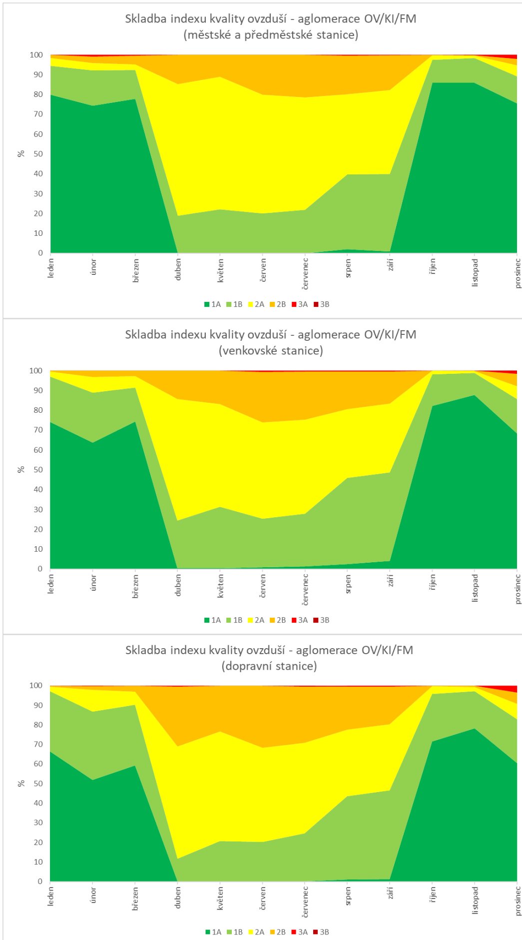
Obrázek 52 - Index kvality ovzduší, aglomerace OV/KI/FM (podle stanic)
