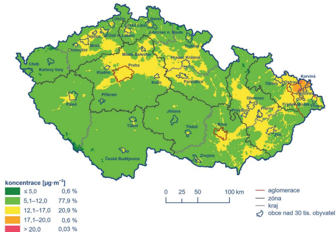
Obrázek 33 - Pole ročních průměrné koncentrace PM 2,5 v roce 2023
