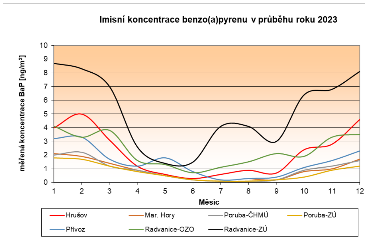
Obrázek 39 Roční chod imisních koncentrací benzo(a)pyrenu v roce 2023 [ng/m 3 ] Okres Ostrava – město
