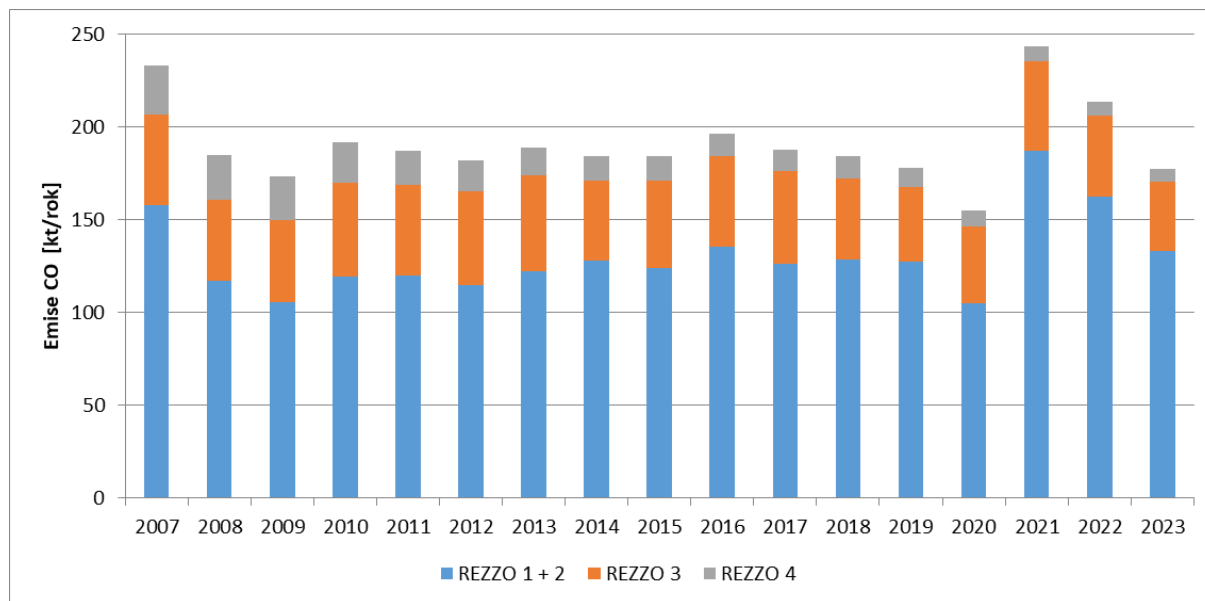
Obrázek 6 - Emise CO jednotlivých skupin zdrojů v MSK
