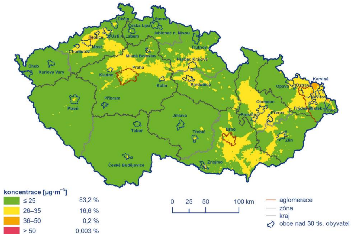
Obrázek 25 – Pole 36. nejvyšší 24-hodinové koncentrace PM 10 v ČR, 2023
