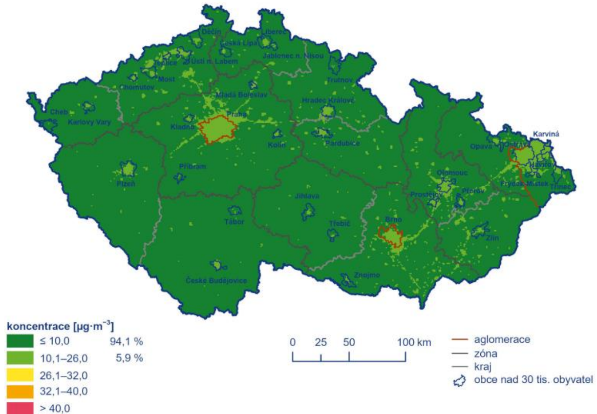
Obrázek 35 - Pole roční průměrné koncentrace \text{NO}_2 v ČR v roce 2023
