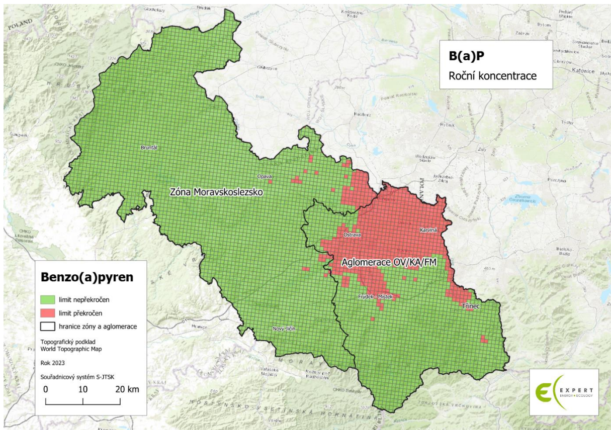
Obrázek 47 - Oblasti s překročením imisního limitu pro roční koncentrace B(a)P - rok 2023
