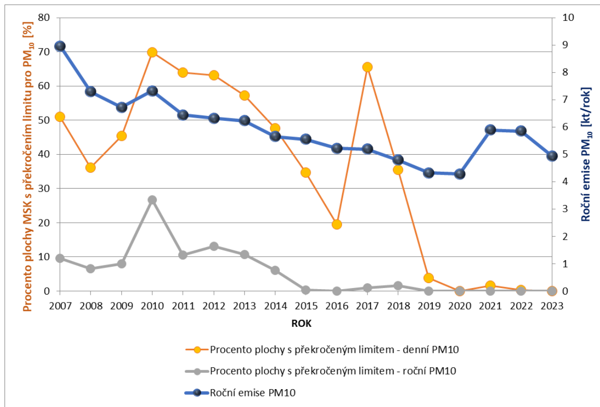
Obrázek 57 - Vyobrazení plochy s překročenými limity a emisí PM 10 v historických datech
