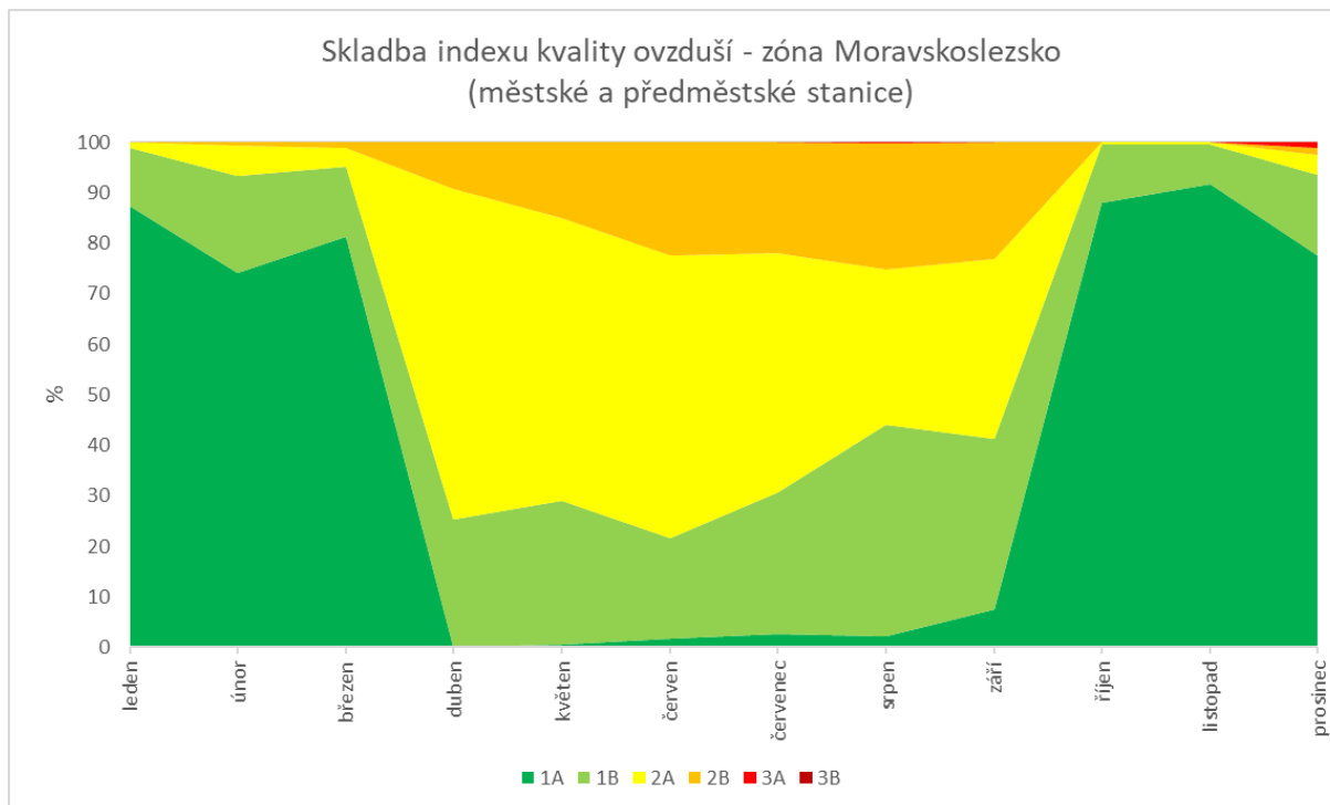
Obrázek 51 - Indexy kvality ovzduší, zóna Moravskoslezsko (podle stanic)
