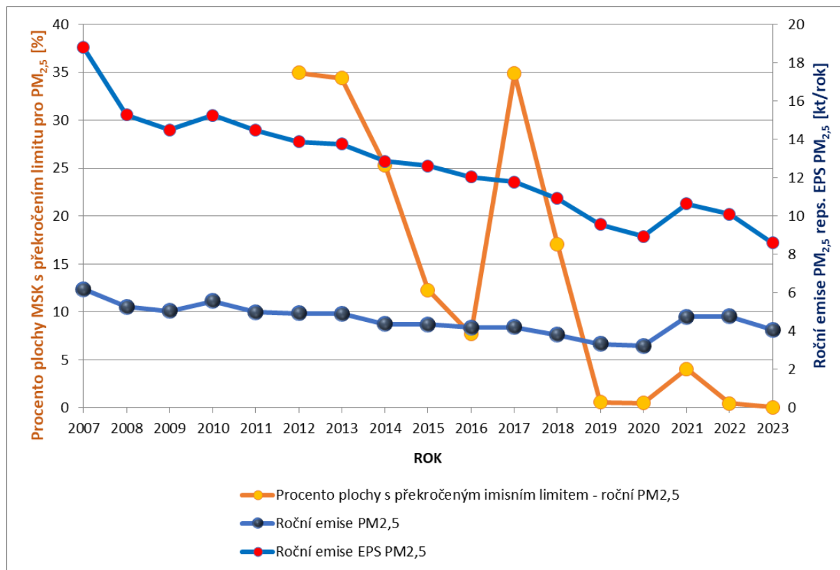
Obrázek 59 - Vyobrazení plochy s překročeným limitem a emisí PM 2,5 v historických datech
