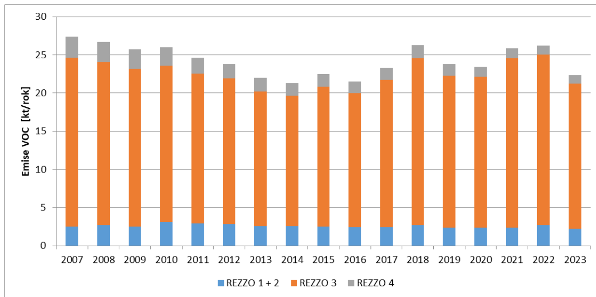
Obrázek 7 - Emise VOC jednotlivých skupin zdrojů v MSK
