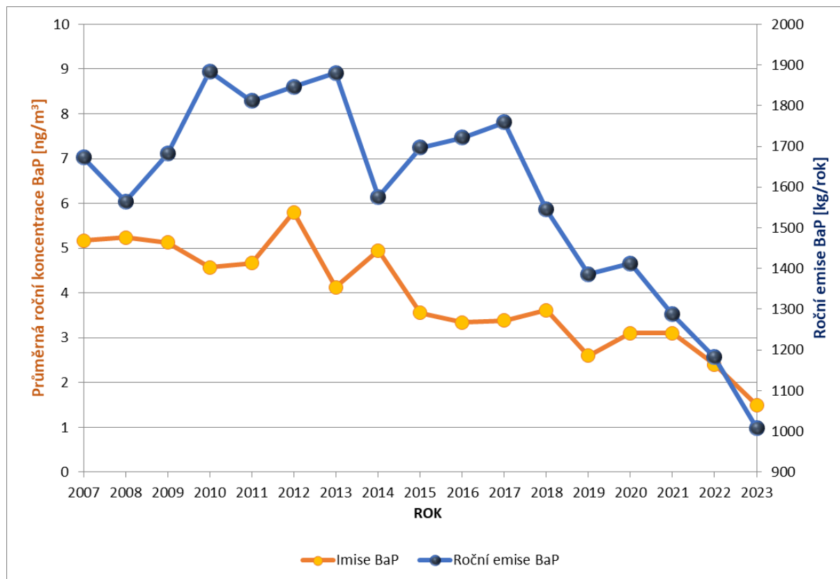
Obrázek 60 - Vyobrazení emisně - imisních vztahů pro BaP
