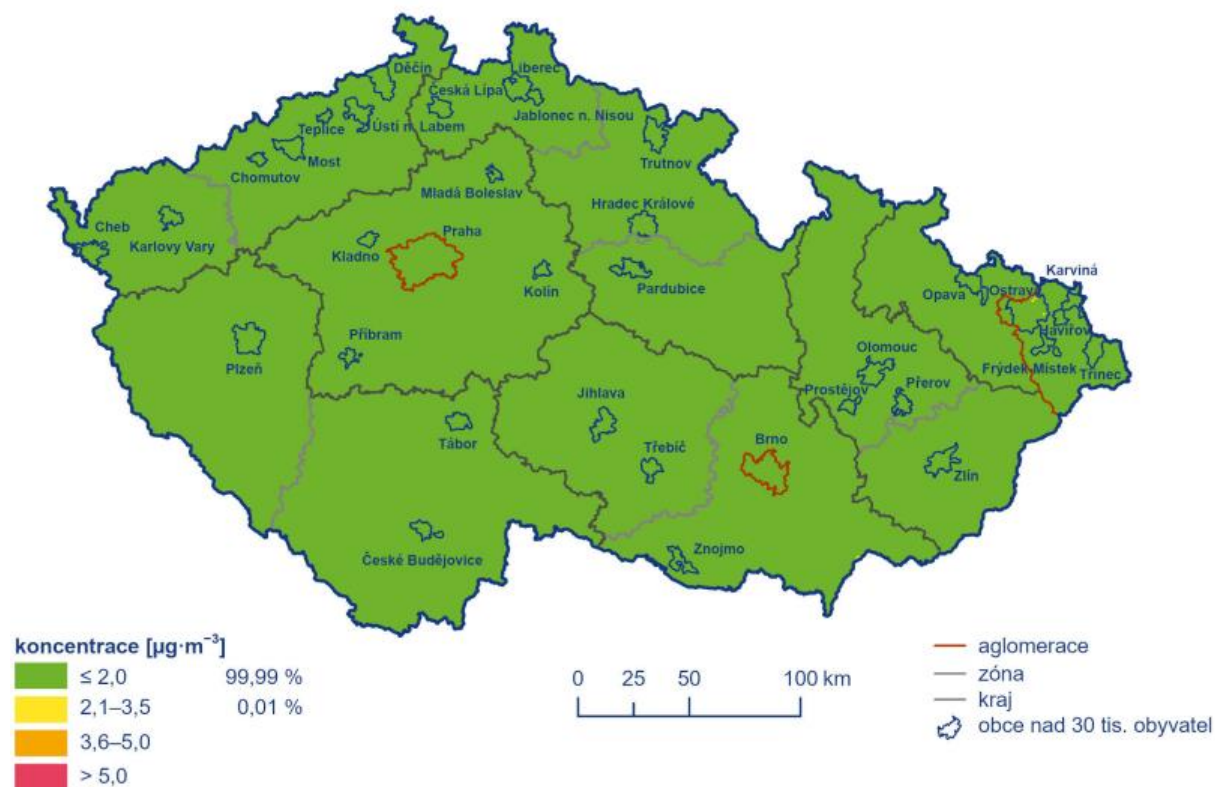
Obrázek 36 - Rozložení průměrné roční imisní koncentrace benzenu v ČR v roce 2023
