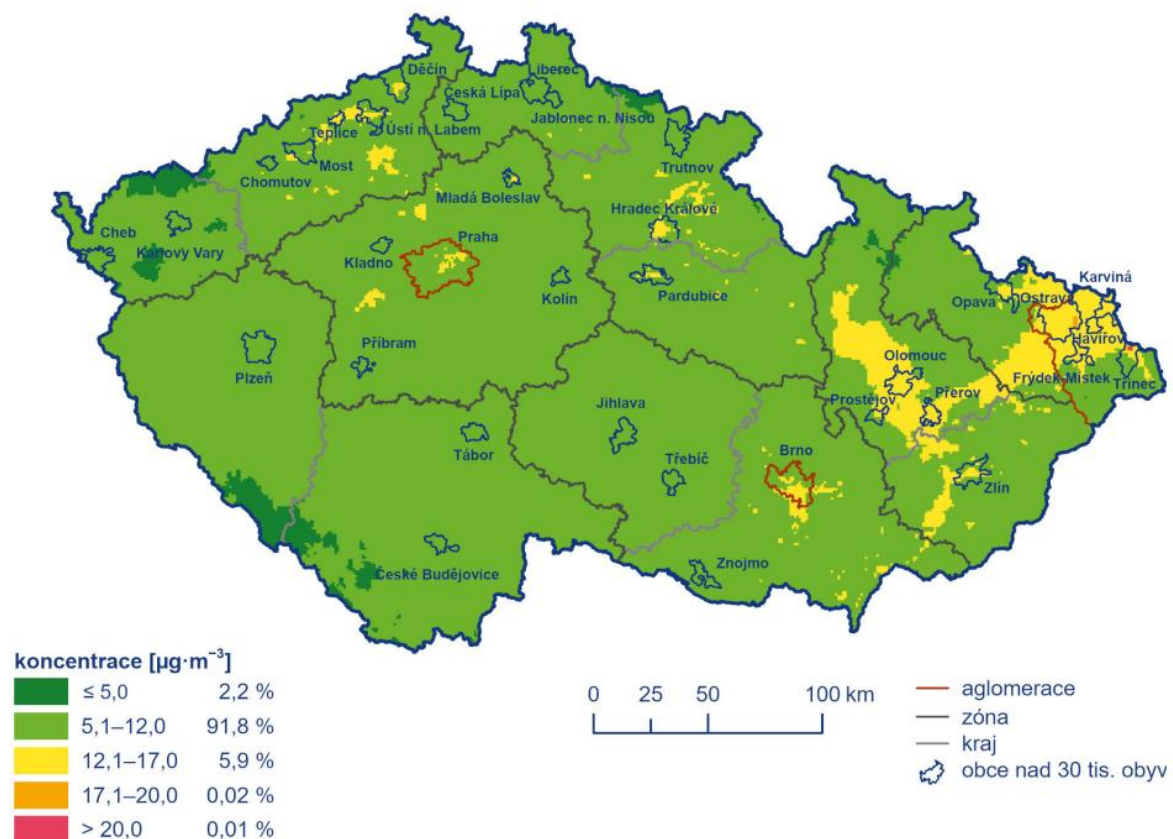
Obrázek 33 - Pole ročních průměrné koncentrace PM 2,5 v roce 2023
