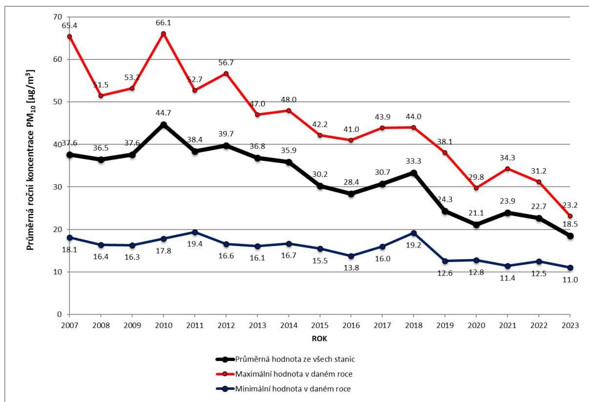
Obrázek 53 – Zobrazení vývoje ročních koncentrací \text{PM}_{10} v rozmezí let 2007 až 2023
