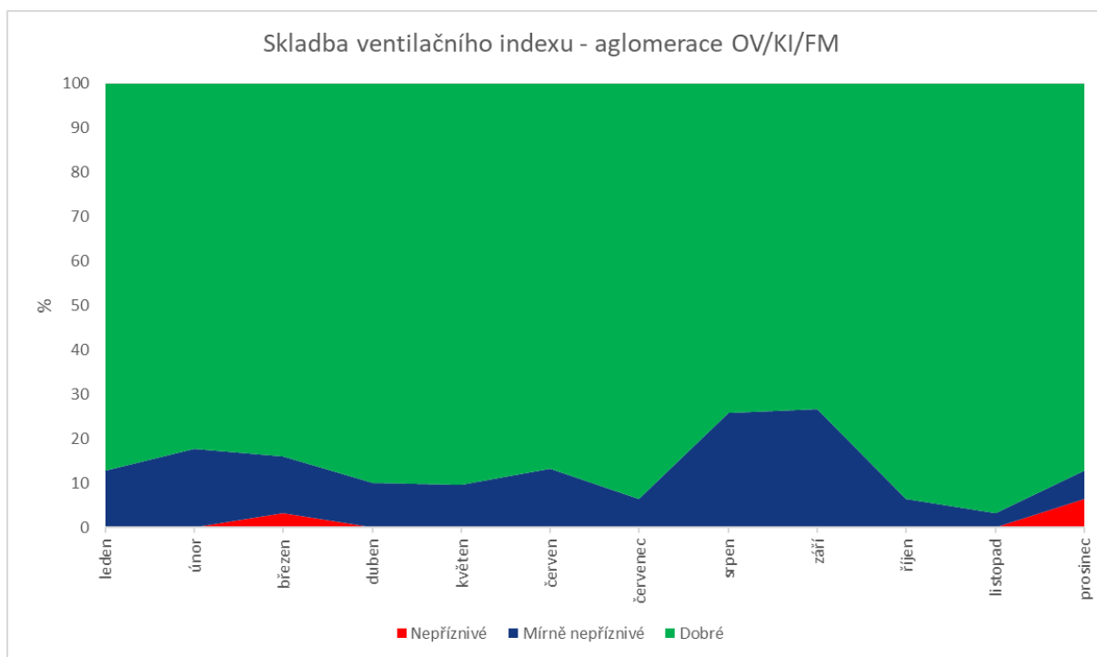
Obrázek 49 - Skladba ventilačního indexu – aglomerace OV/KI/FM
