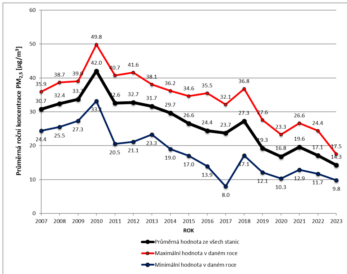
Obrázek 54 – Zobrazení vývoje ročních koncentrací PM 2,5 v rozmezí let 2007 až 2023
