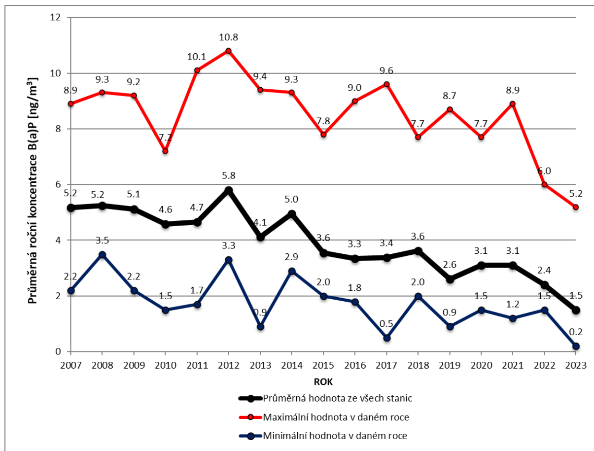
Obrázek 55 – Zobrazení vývoje ročních koncentrací benzo(a)pyrenu v rozmezí let 2007 až 2023
