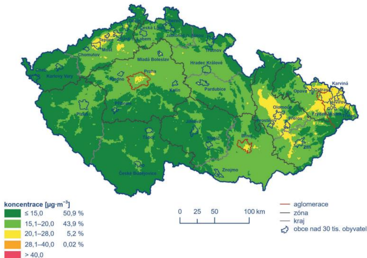
Obrázek 27 - Rozložení průměrné roční imisní koncentrace PM 10 v ČR v roce 2023
