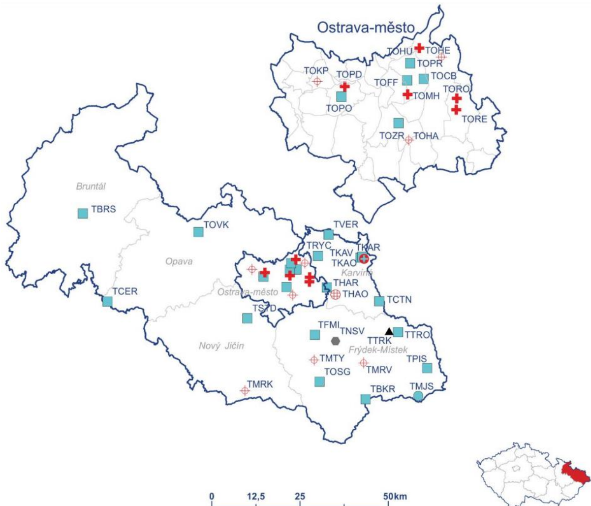
Obrázek 19 - Síť imisního monitoringu na území Moravskoslezského kraje v roce 2023
