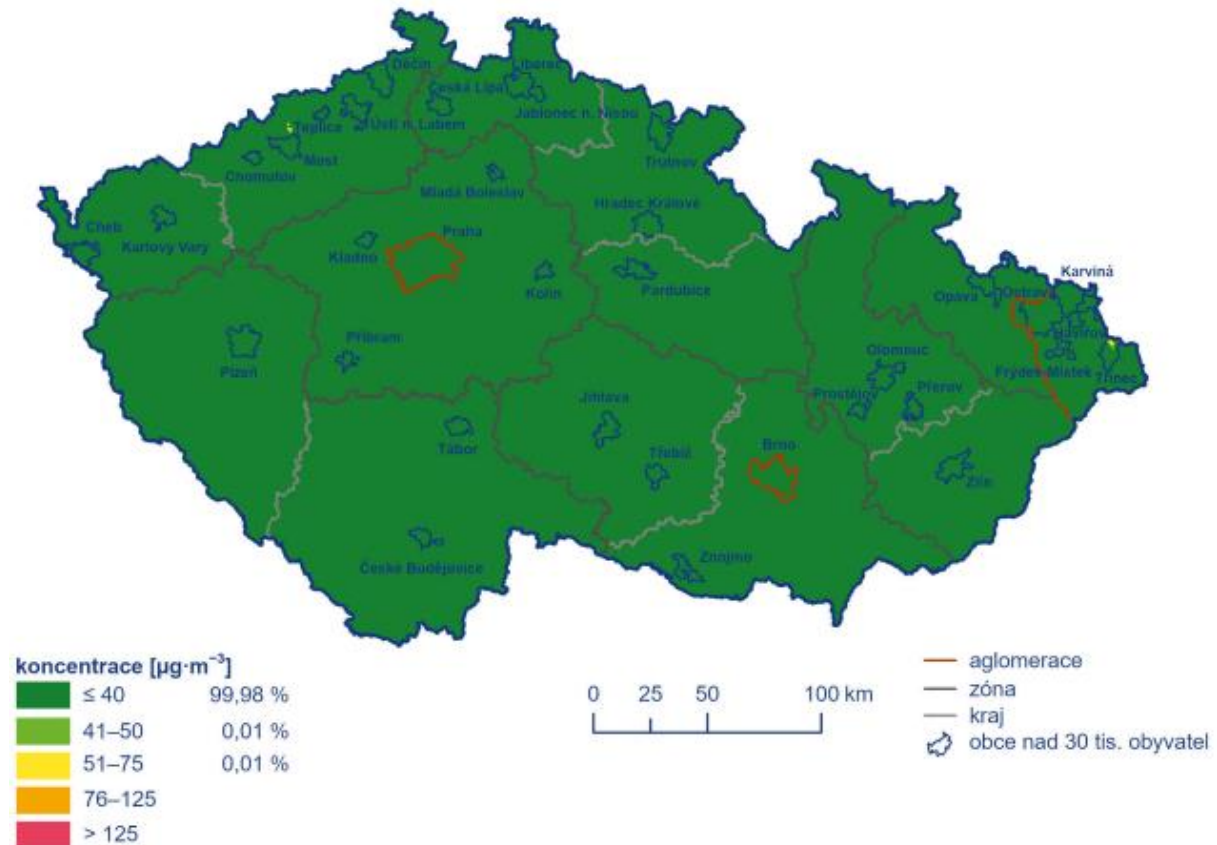
Obrázek 34 - Pole 4. nejvyšší 24hodinové koncentrace SO 2 v roce 2023
