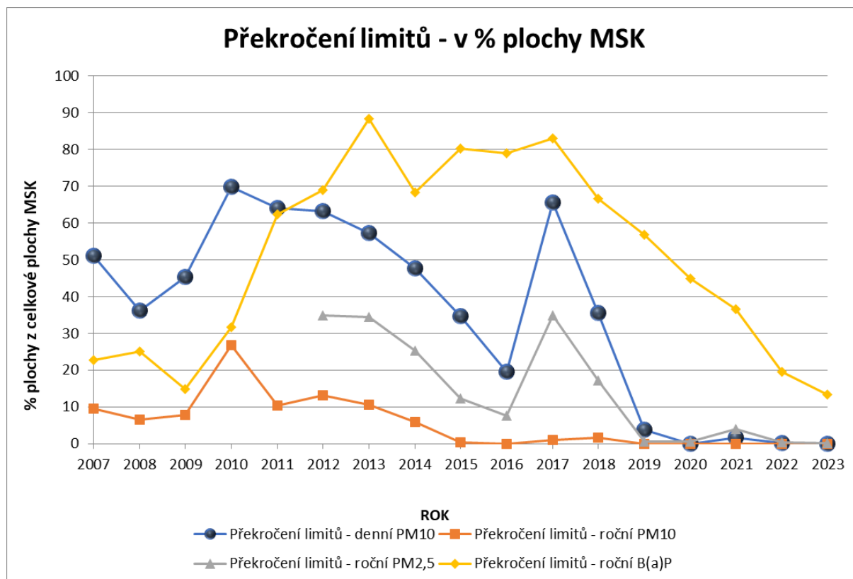
Obrázek 62 - Grafické vyhodnocení procenta plochy s překročenými limity na ploše MSK
