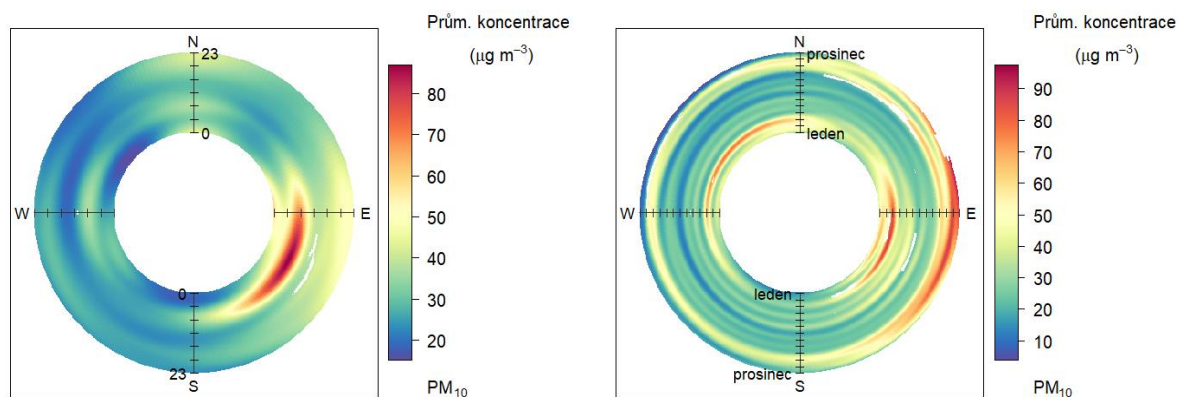
Obr. 30– Denní a roční chod koncentrací PM 10 , lokalita Ostrava – Mariánské Hory, rok 2018
