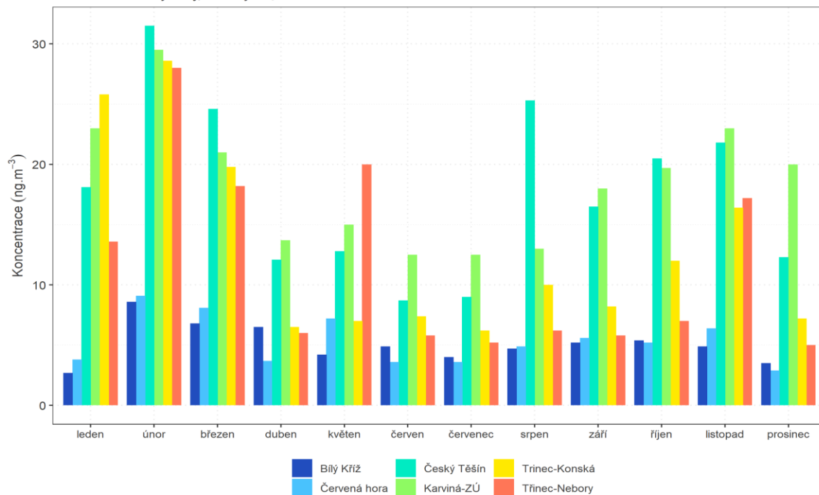
Graf 30: Roční chod imisních koncentrací olova – okres Karviná, Frýdek-Místek a Opava Průměrné měsíční koncentrace Pb Moravskoslezský kraj, okresy Frýdek - Místek, Karviná a Opava, rok 2018
