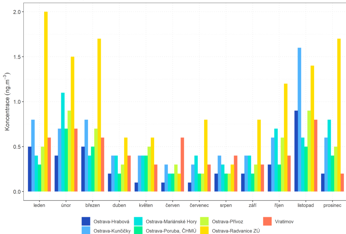
Graf 35: Roční chod imisních koncentrací kadmia - okres Ostrava-město, rok 2018
