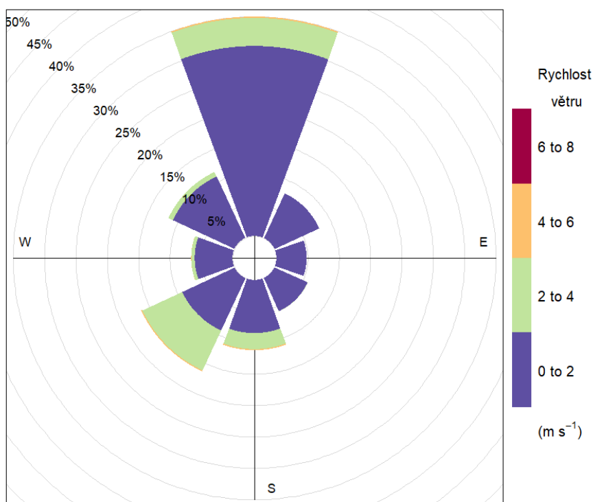
Obr. 17 – Větrná růžice členěná dle rychlosti větru, Ostrava – Radvanice, rok 2018
