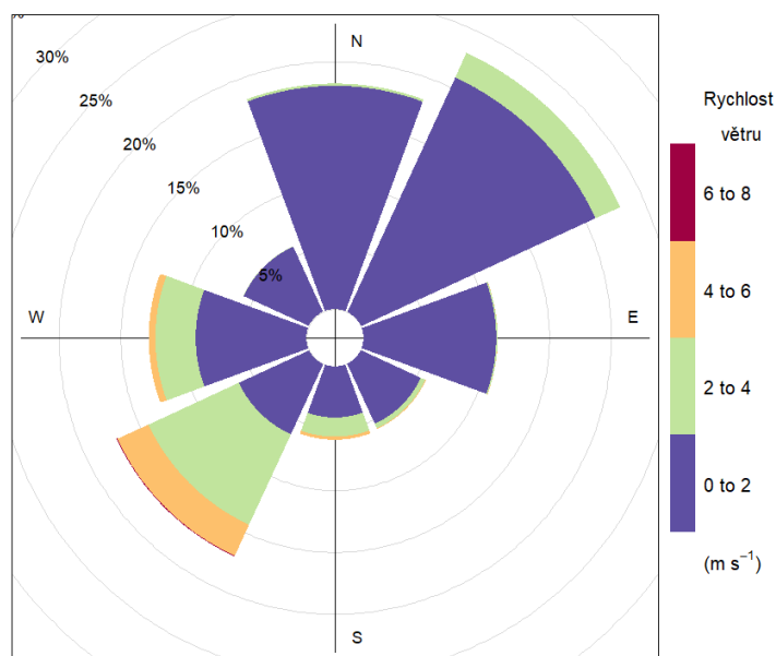
Větrná růžice členěná dle rychlosti větru
