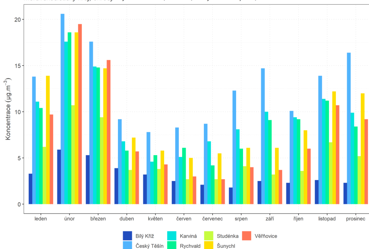
Graf 21: Roční chod imisních koncentrací \text{SO}_2
