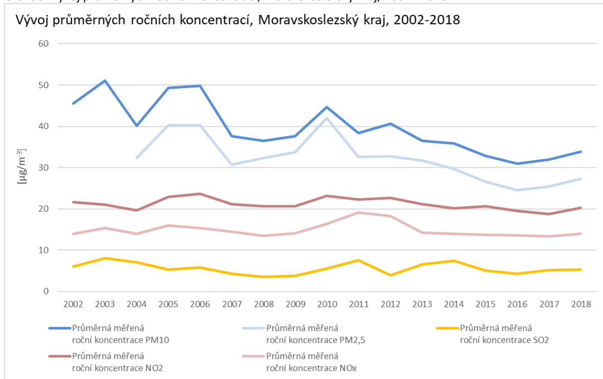
Graf 38: Vývoj průměrných ročních koncentrací, Moravskoslezský kraj, 2002 - 2018
